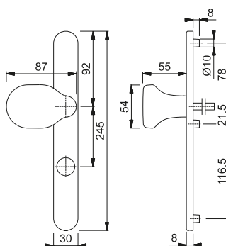
bouton E86G
