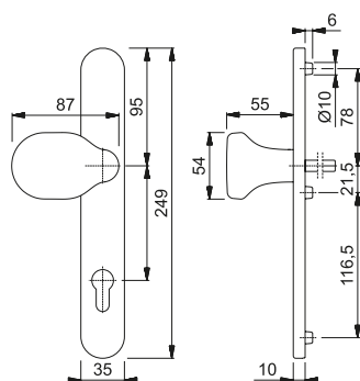
bouton E86G
