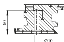
profilé Pural
